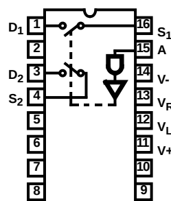
DPST HI-5044 (50Ω)
