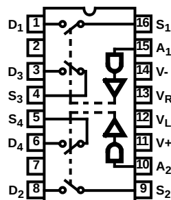
DUAL DPST HI-5045 (50Ω), HI-5049 (25Ω)
