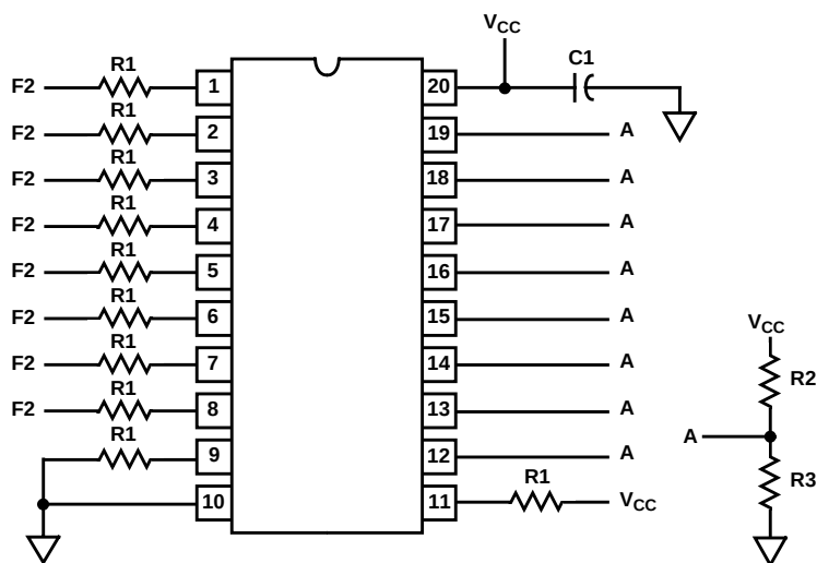
MD82C87H Cerdip
