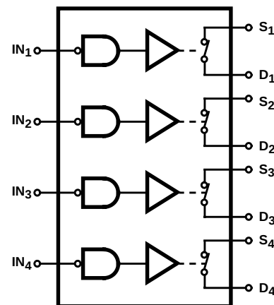
DG202
