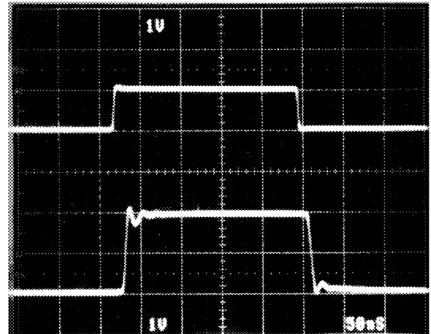
Vertical Scale: V_{IN} = 1\text{V}/\text{Div.} , V_{OUT} = 1\text{V}/\text{Div.} Horizontal Scale: 50\text{ns}/\text{Div.}
