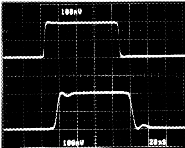
Vertical Scale: V_{IN} = 100\text{mV}/\text{Div.} , V_{OUT} = 100\text{mV}/\text{Div.} Horizontal Scale: 20\text{ns}/\text{Div.}
