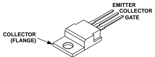
JEDEC TO-220AB
