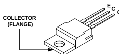
JEDEC TO-220AB
