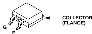
JEDEC TO-263AB
