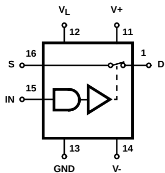
DIP (JE, PE) SPST IH5140
