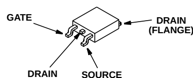
JEDEC TO-252AA
