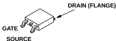
JEDEC TO-252AA
