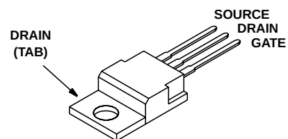
JEDEC TO-220AB
