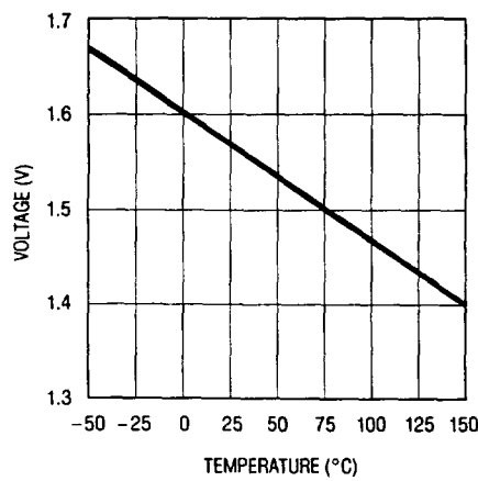
Enable Threshold
