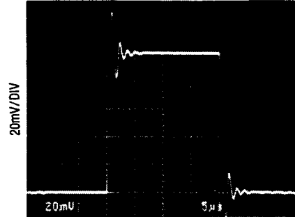
A_V = +1 , C_{LOAD} = 1000pF , 5\mu s/DIV
