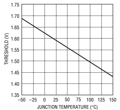
Enable Threshold
