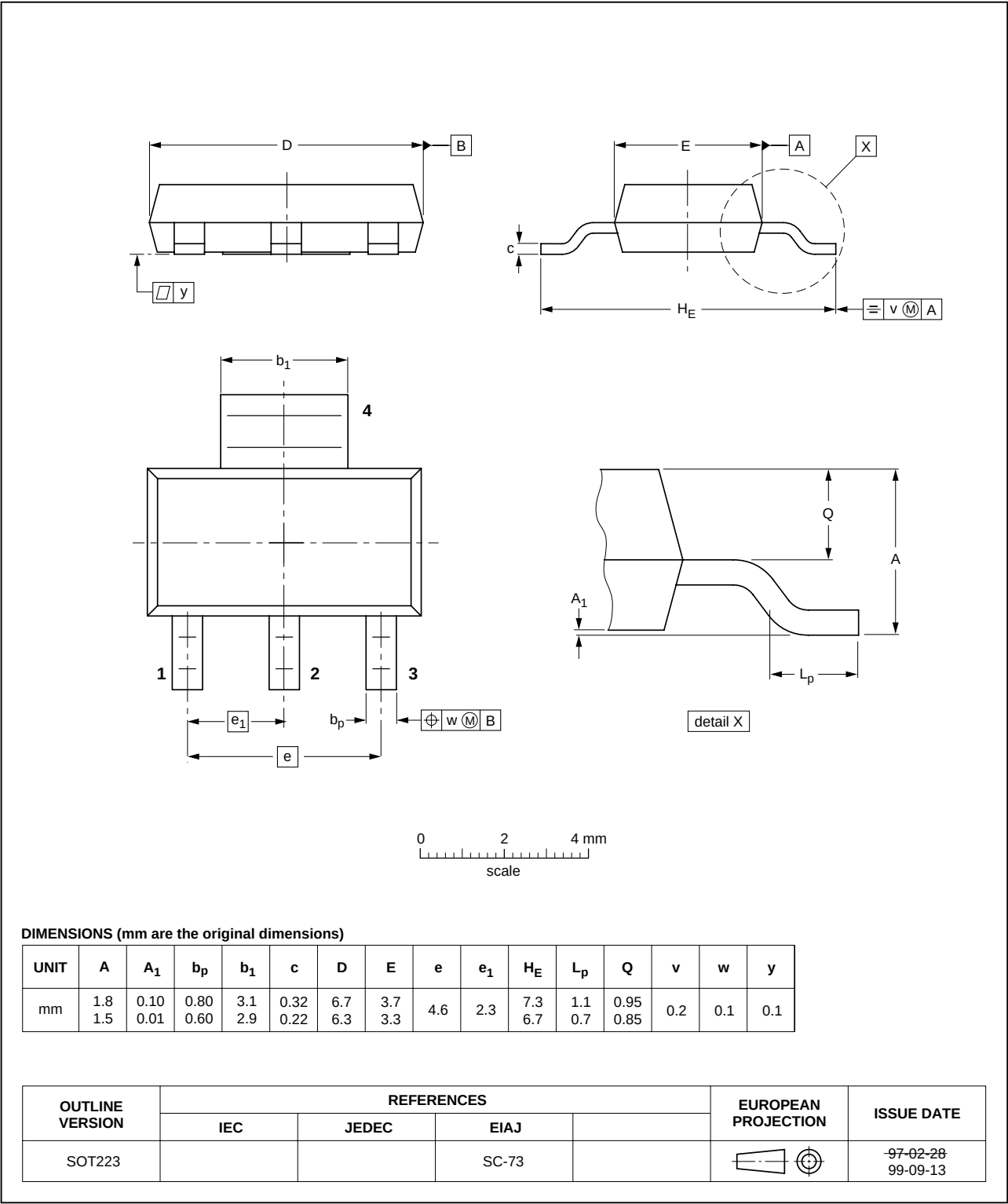
Fig 15. SOT223.
