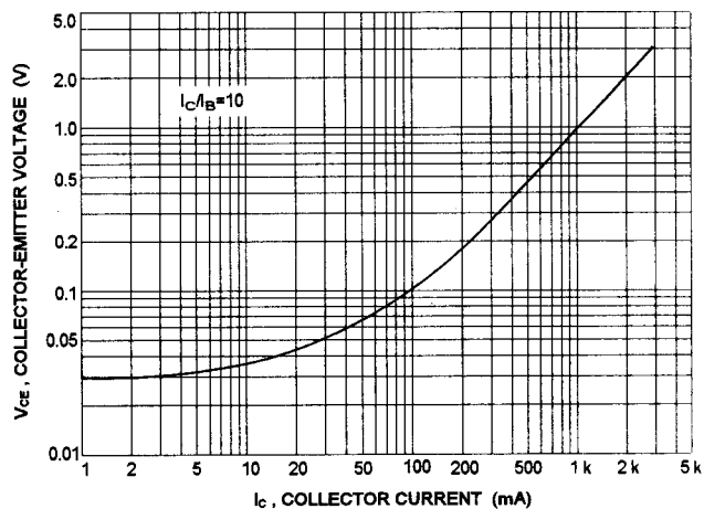
V_{CE} - I_C
