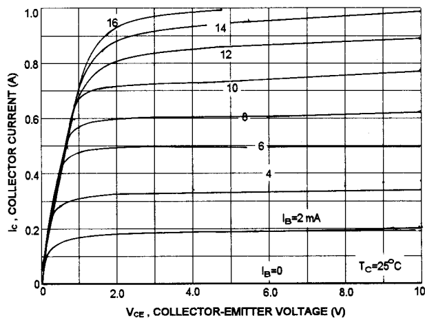
I_C - V_{CE}
