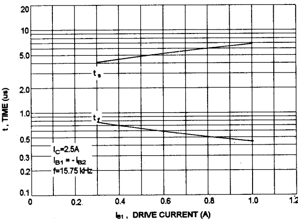
t_s, t_f - I_{B1}
