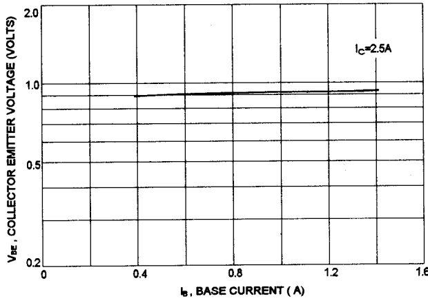
V_{BE(SAT)} - I_B
