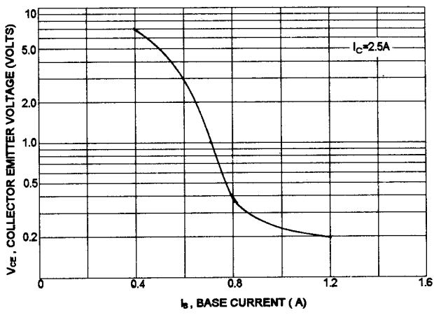
V_{CE(SAT)} - I_B
