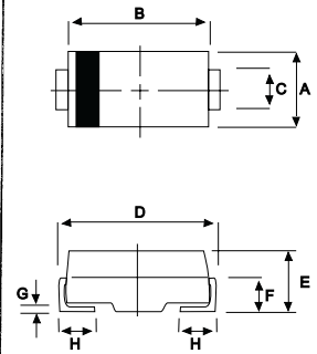
DO-214AC(SMA)
