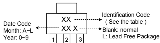
(4) SOT89-3L
