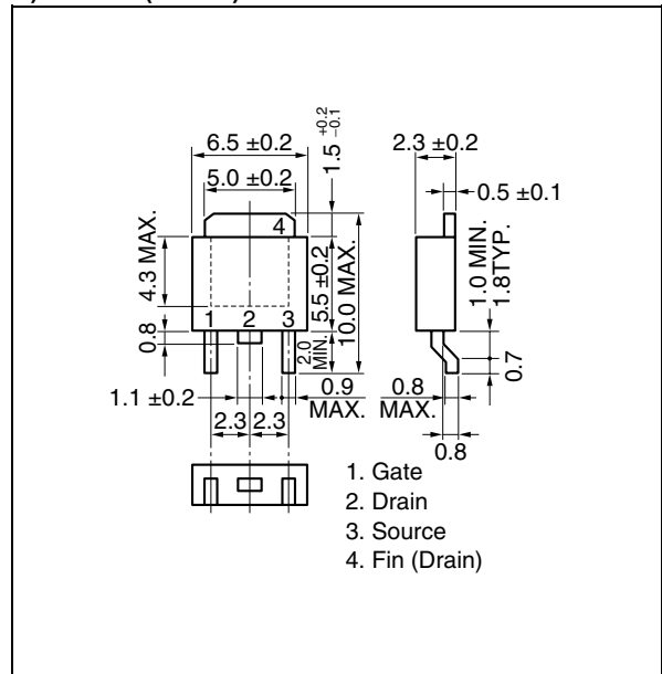
2) TO-252 (MP-3Z)
