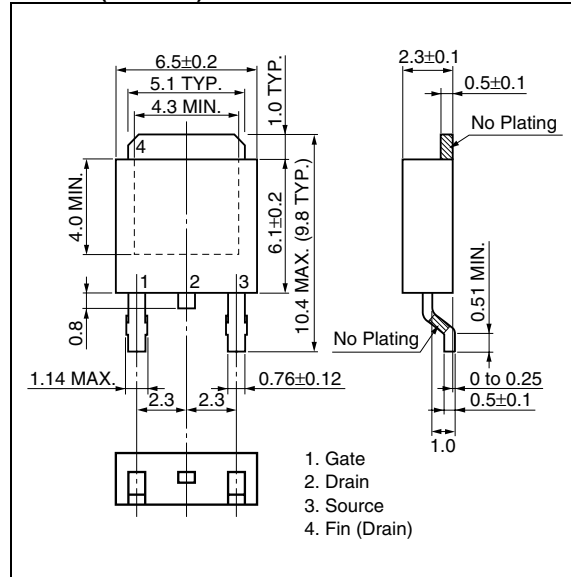
TO-252 (MP-3ZK)
