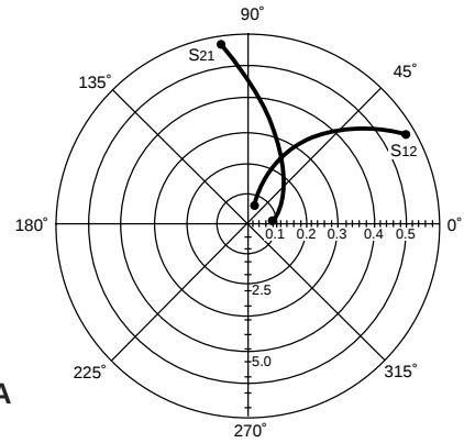
NE97833 VCE = -8 V, IC = -10 mA
