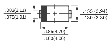
SMB (DO-214AA)
