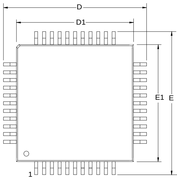
44 PIN TQFP
