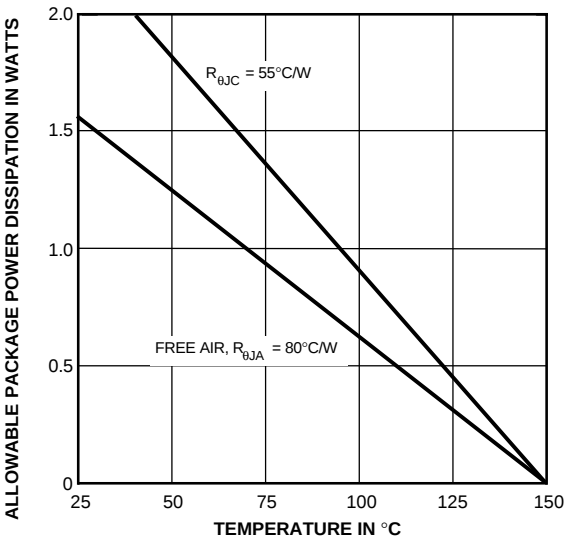
Dwg. GP-009-1B
