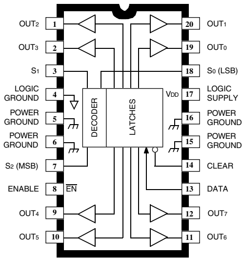
A6A259KA (DIP)
