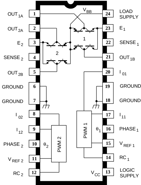
UDN2916B (DIP)
