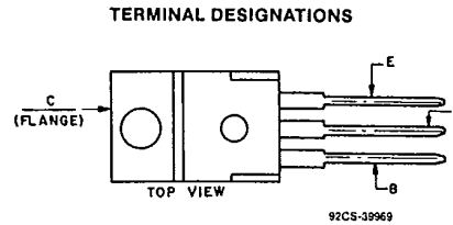
JEDEC TO-220AB
