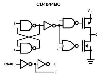
CD4044BC
