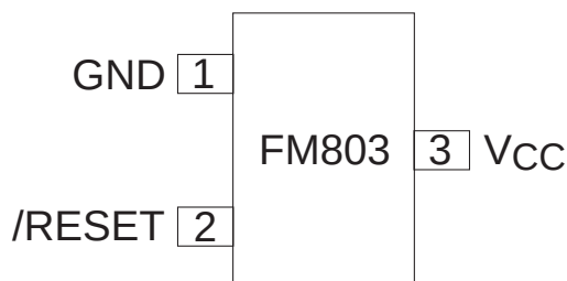
SC70-3 & SOT23-3 Packages
