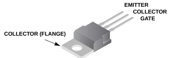
JEDEC TO-220AB
