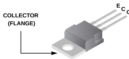
JEDEC TO-220AB
