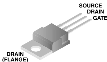
JEDEC TO-220AB
