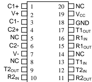
20-Pin TSSOP
