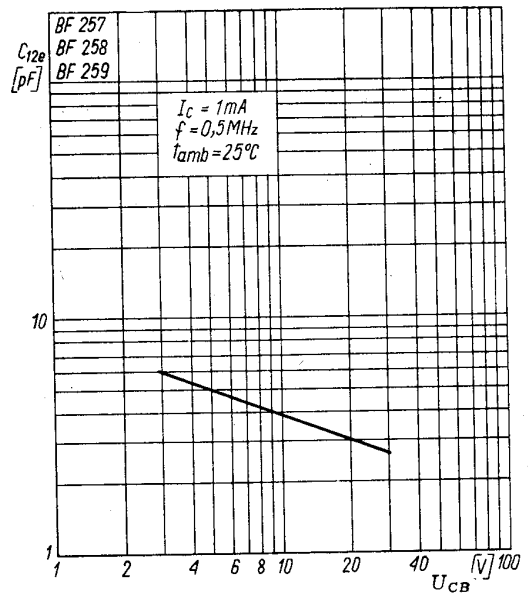
Zależności pojemności sprzężenia zwrotnego C_{12e} od napięcia U_{CB} ; C_{12e} = f(U_{CB})
