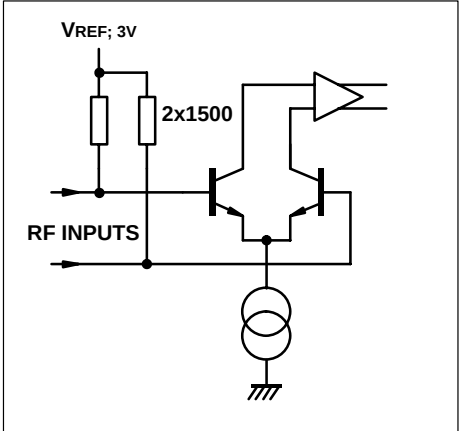
RF inputs
