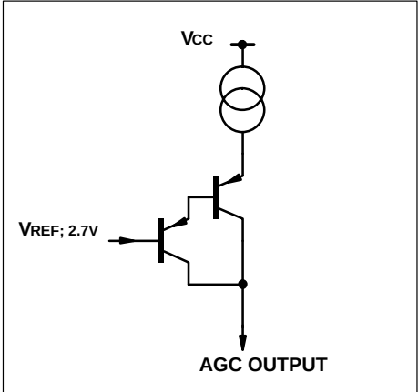
AGC output
