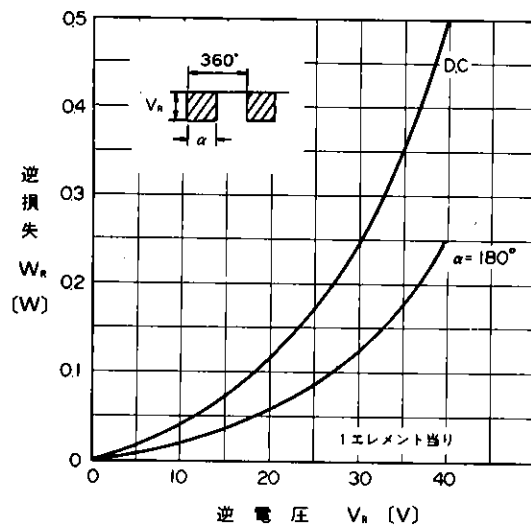
逆損失特性 Reverse Power Dissipation
