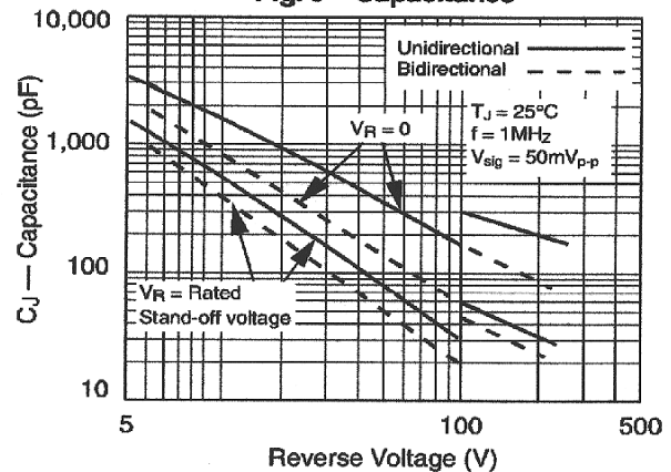
Fig. 6 – Capacitance
