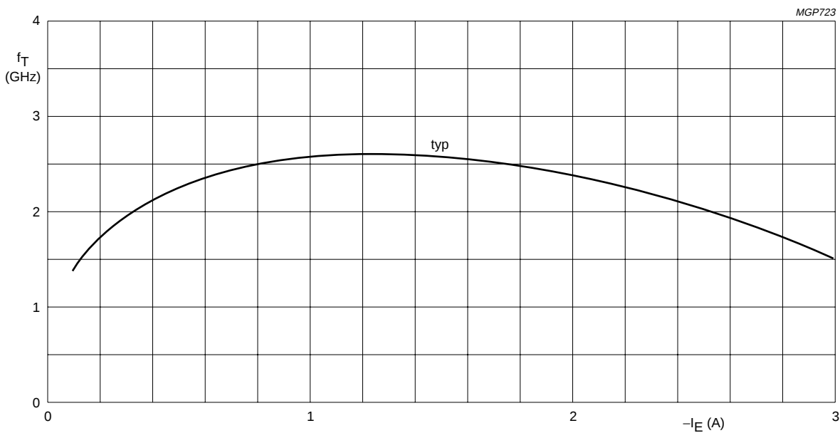
Fig.8 V_{CB} = 25\text{ V} ; f = 500\text{ MHz} ; T_j = 25\text{ }^{\circ}\text{C} .
