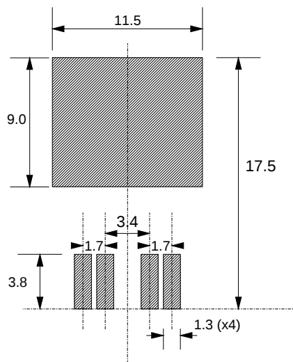
Fig.34. SOT426
