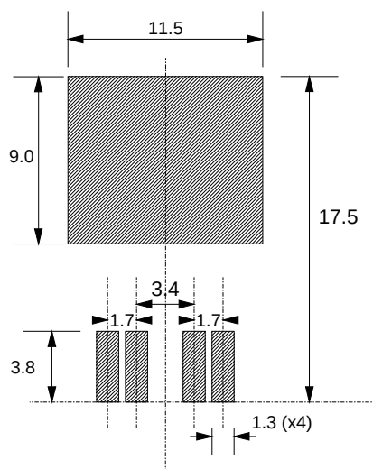
Fig.39. SOT426
