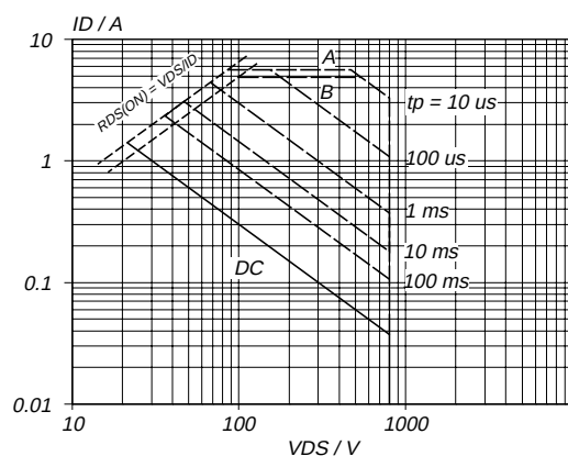
Fig.3. Safe operating area. T_{hs} = 25^\circ\text{C} I_D & I_{DM} = f(V_{DS}) ; I_{DM} single pulse; parameter t_p
