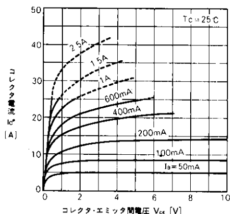
出力特性
