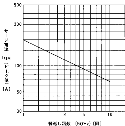
繰返し回数 (50Hz) (回) サージ電流耐量 Surge Capability
