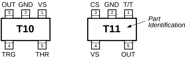
SOT-23-5 (M5)
