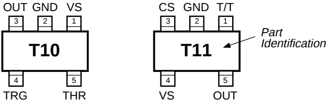
SOT-23-5 (M5)
