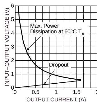
Si4433DY SOA
