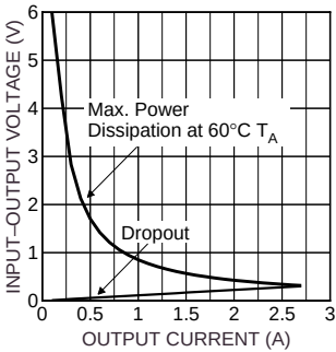
Si3445DV SOA
