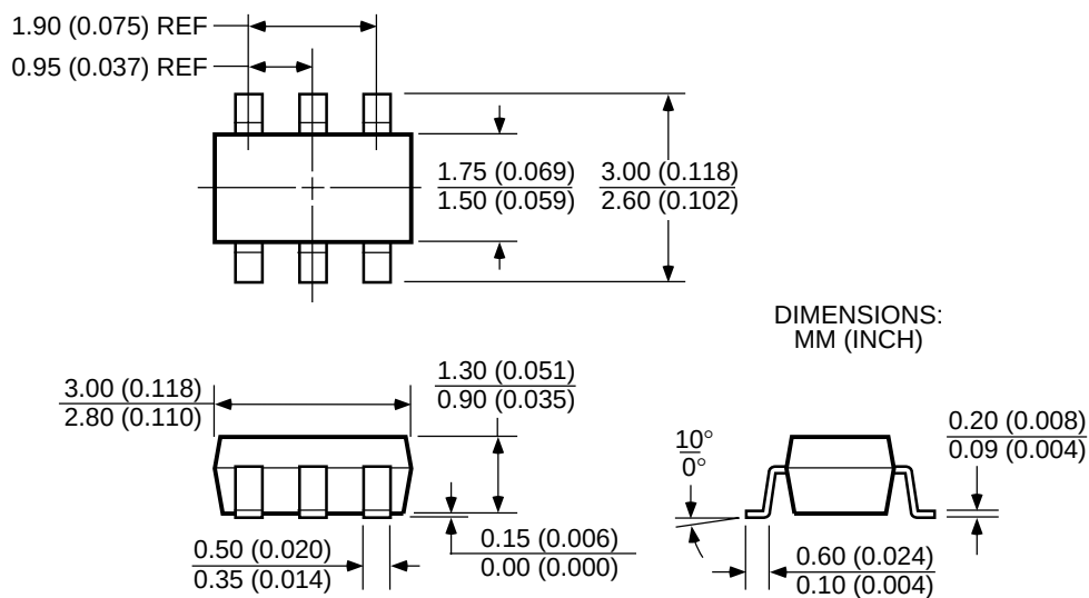
SOT-23-6 (M6)
