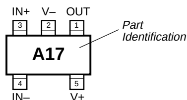
SOT-23-5 (M5)
