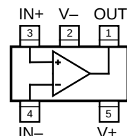
SOT-23-5 (M5)
