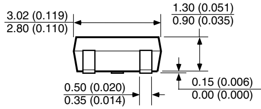
SOT-23-5 (M5)
