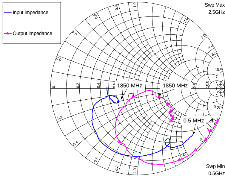
1900MHz LNA
