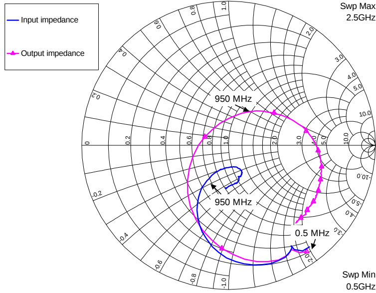
900MHz LNA
